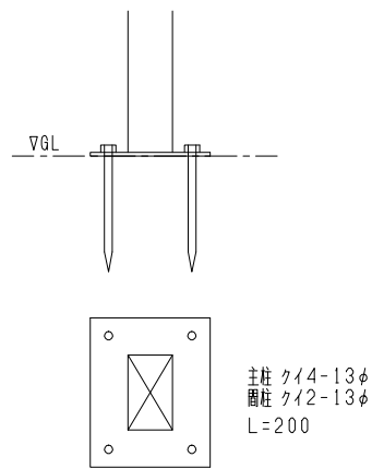
主柱ベース図 S = 1 / 10
