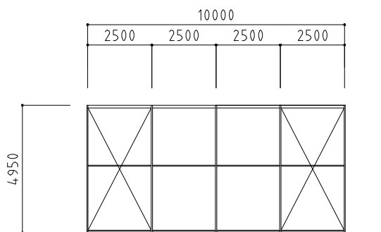
軸組図 S = 1 / 150
