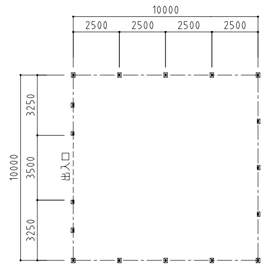
平面図 S = 1 / 150
