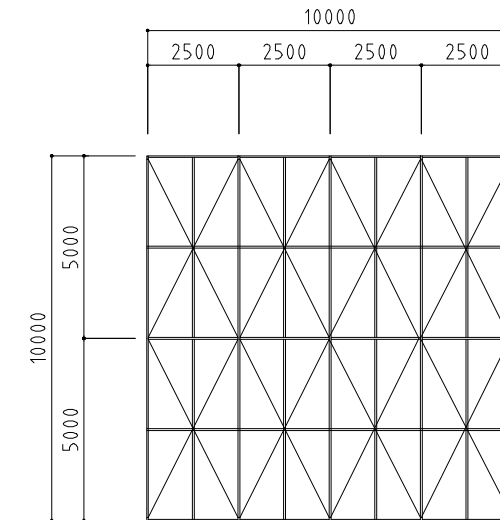
梁伏図 S = 1 / 150
