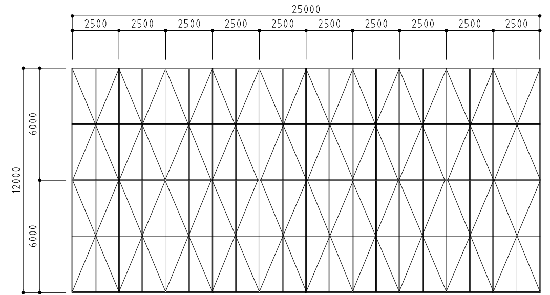
梁伏図 S = 1 / 150
