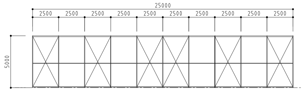
軸組図 S = 1 / 150
