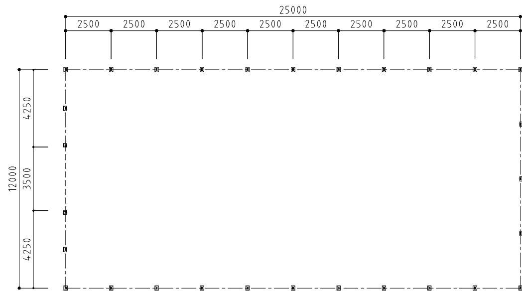
基礎伏図 S = 1 / 150
